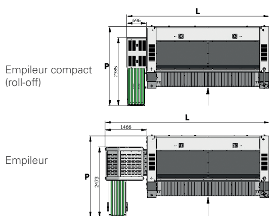
Empileur compact
